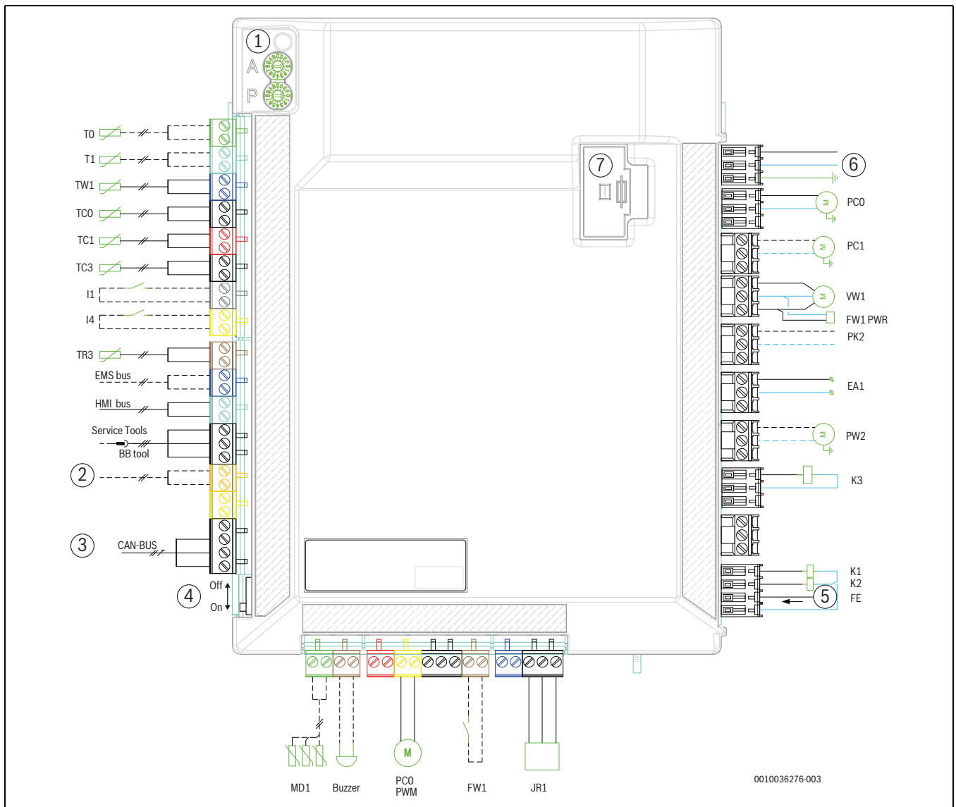
35. ábra A beltéri egység telepítési modulja
