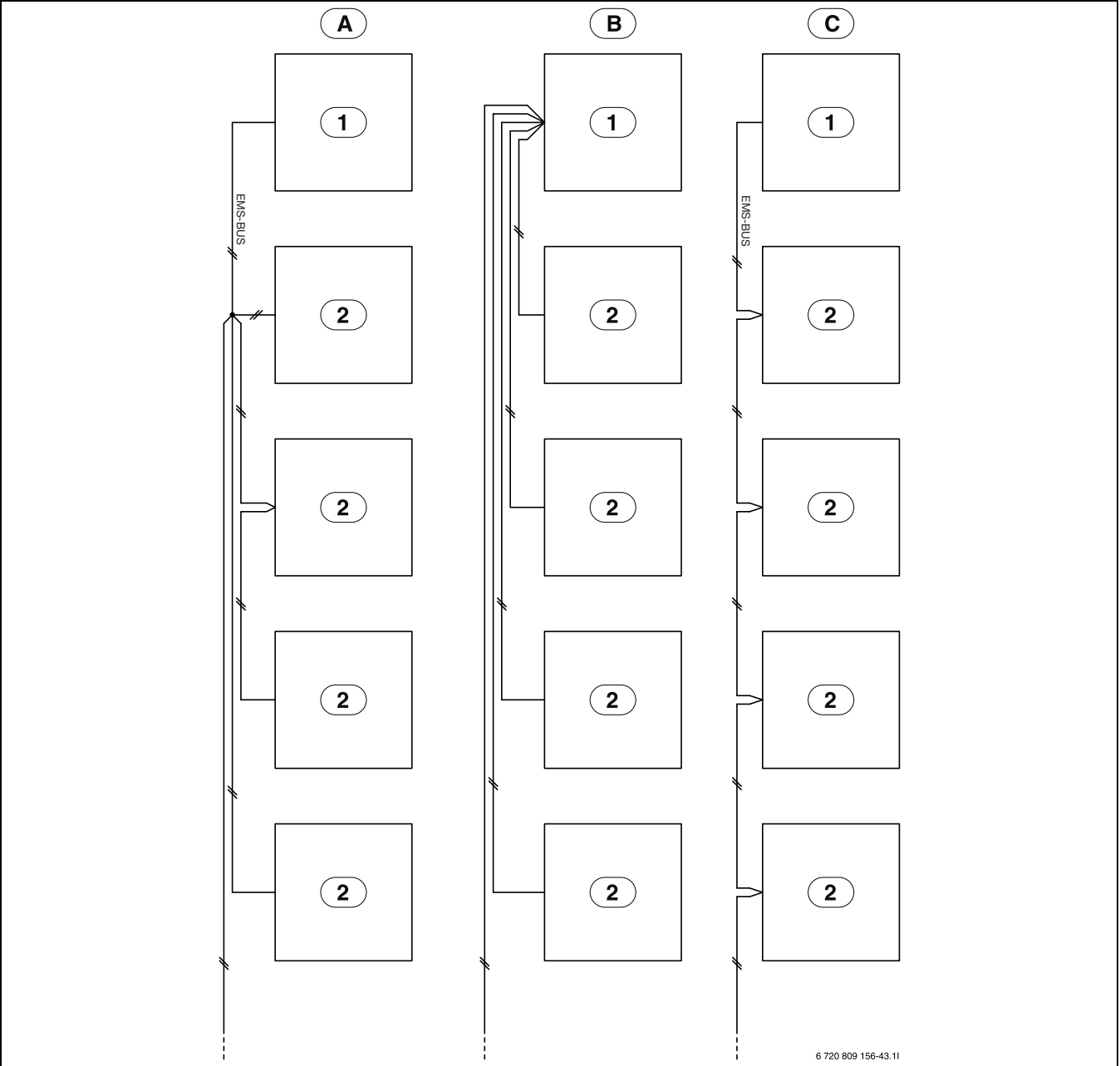
42. ábra Alternatív csatlakoztatás az EMS-BUS-hoz
