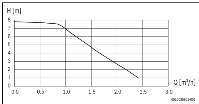
28. ábra Aprimer keringtető szivattyú (PC0) kapacitásgörbéje
