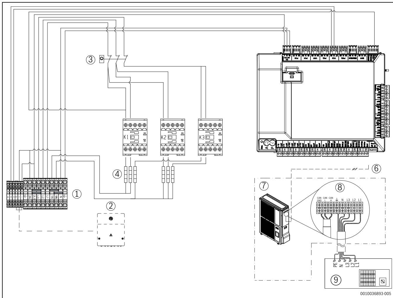
41. ábra 400 V, 3N~ beltéri egység, 400 V, 3N~ kültéri egységgel
