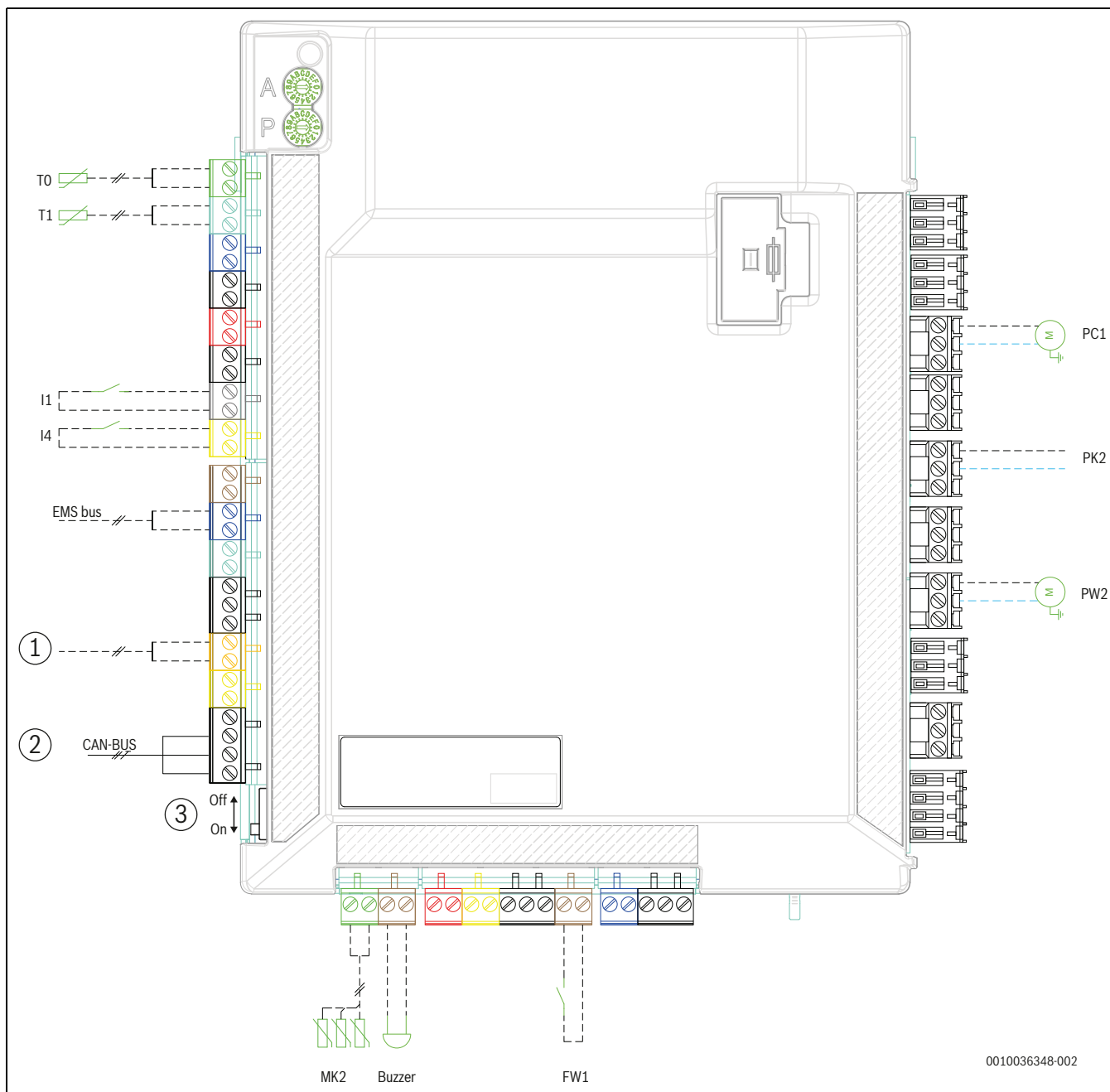
12. ábra A beltéri egység telepítési modulja
