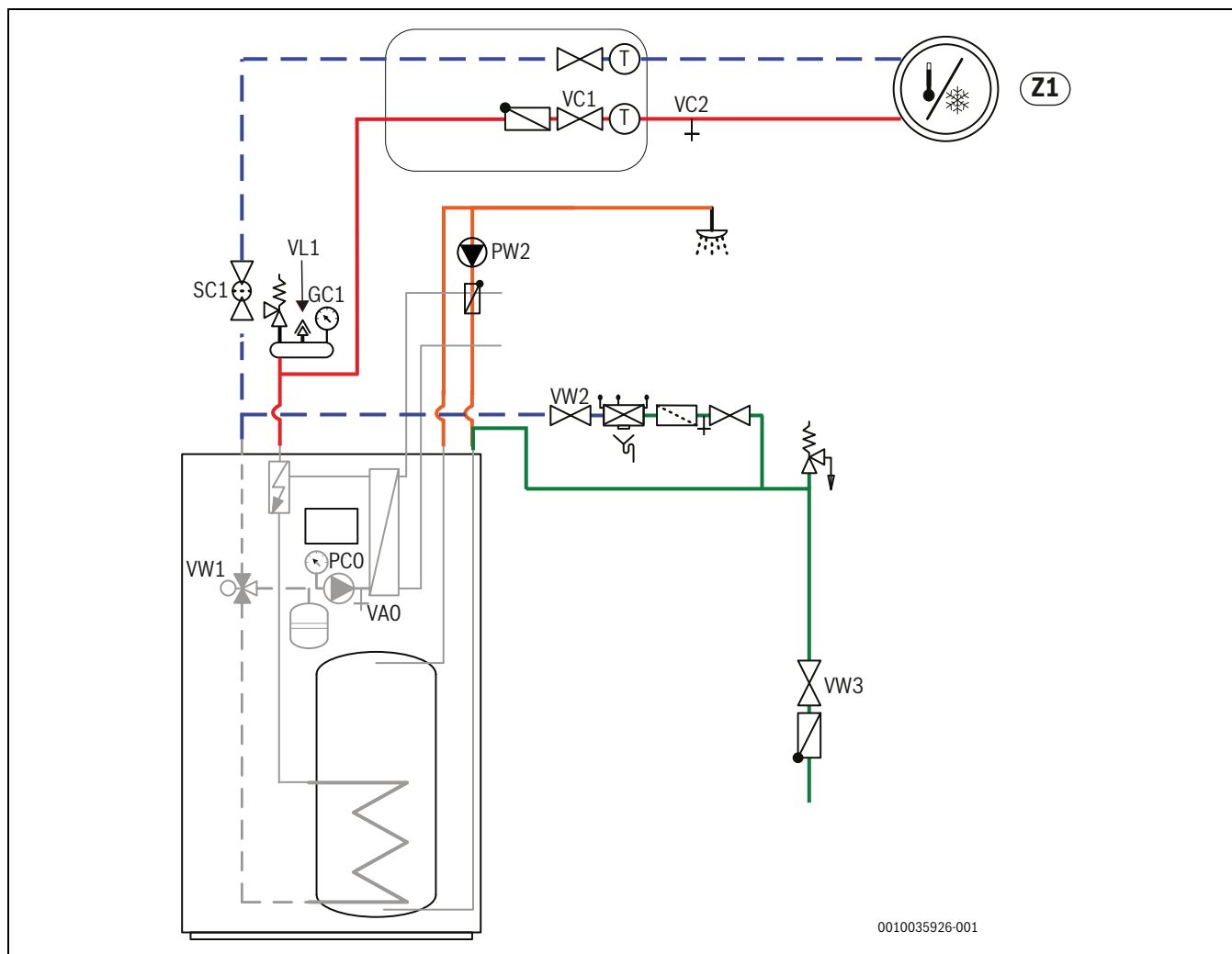
17. ábra A beépített elektromos fűtéstápegítéssel ellátott beltéri egység légtelenítése
