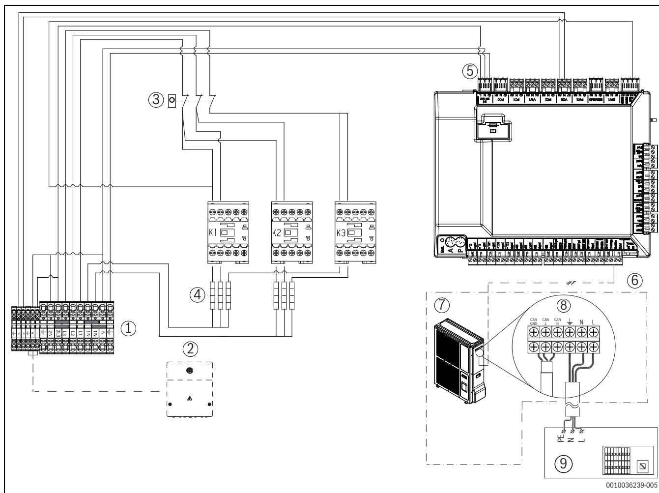
40. ábra 400 V 3N~ beltéri egység, 230 V~ kültéri egységgel
