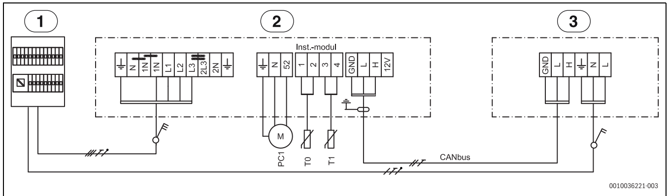
38. ábra Kapcsolási rajz – 9 kW, 3N~
