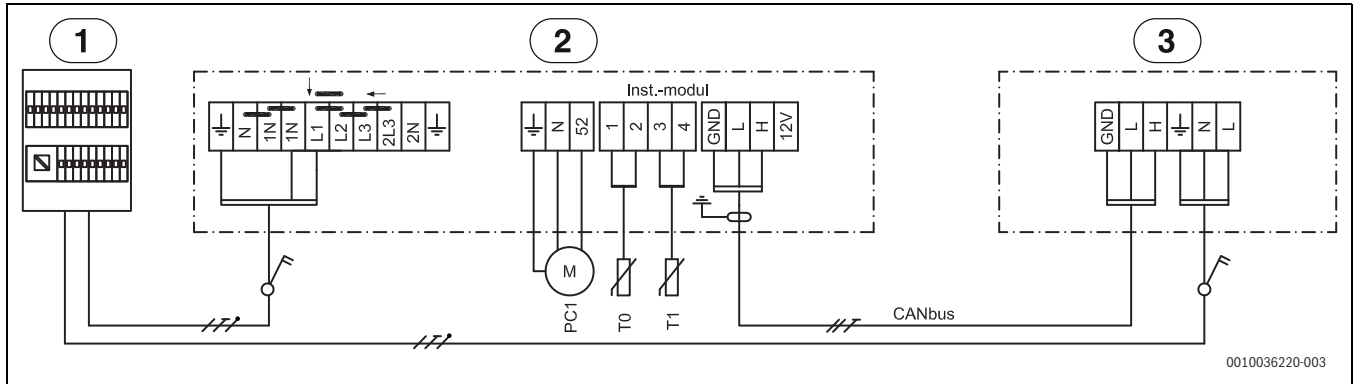
37. ábra Kapcsolási rajz – 9 kW, 230 V~
