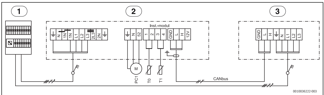
39. ábra Kapcsolási rajz – 9 kW, 400 V, 3N~, másfajta kábelezés
