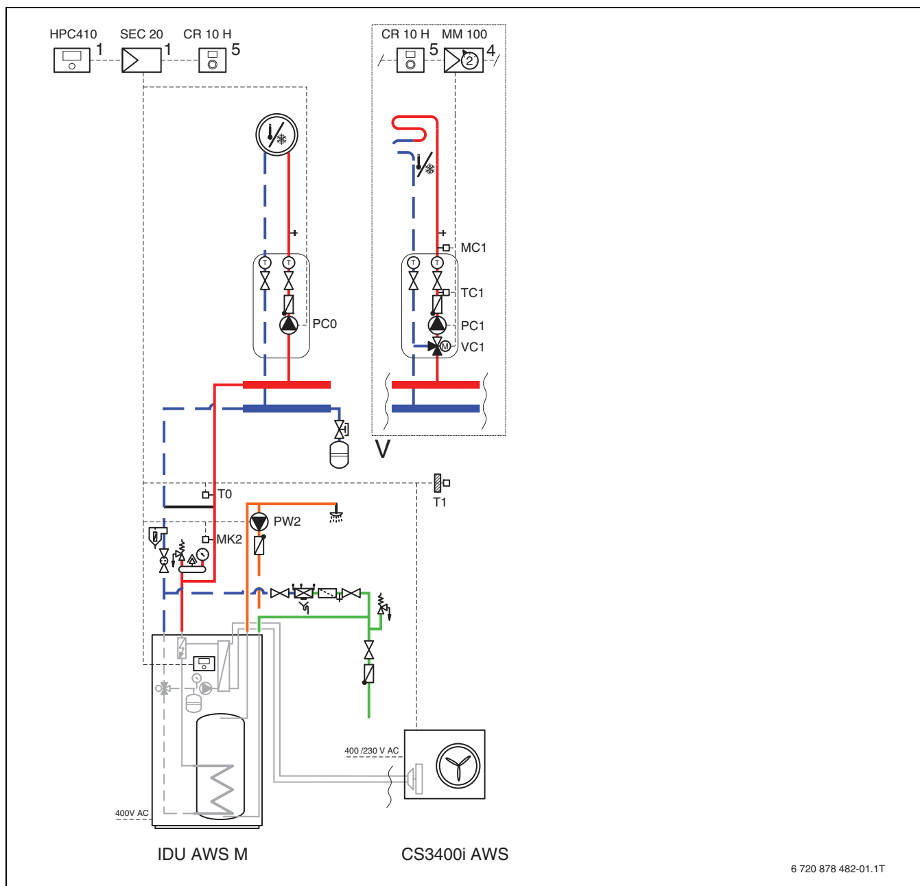
33. ábra Kültéri egység beltéri egységgel és egy vagy több fűtőkörrel
